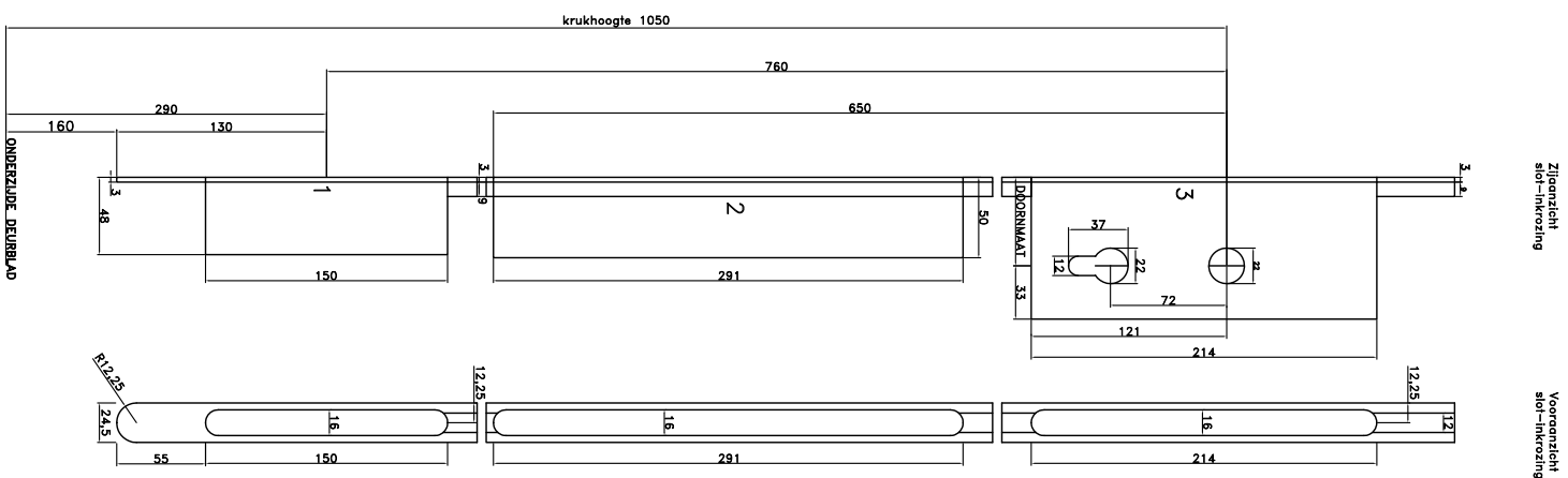
VOORBEELD DETAL 1: deurdikte 38 / 54 mm T-groef
