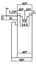
T-GROEF: * Bij afwijkende deurdiktes / details dienen de maten met een * herberekend te worden
